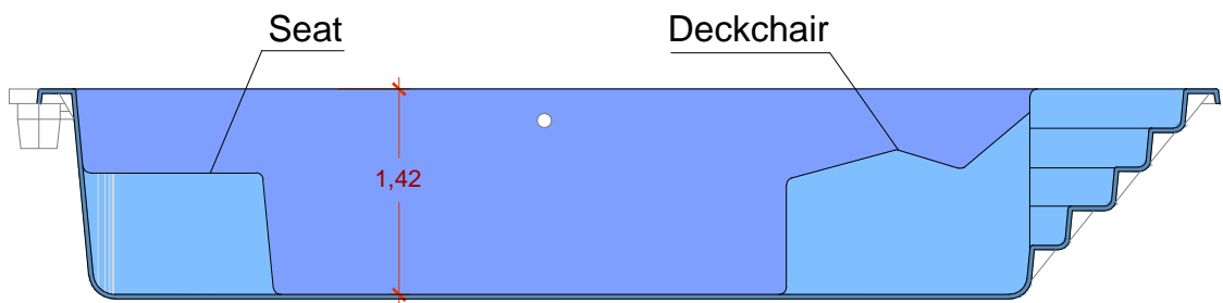
LONGITUDINAL SECTION
